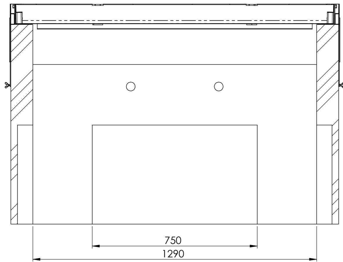
SCHNITT B-B
