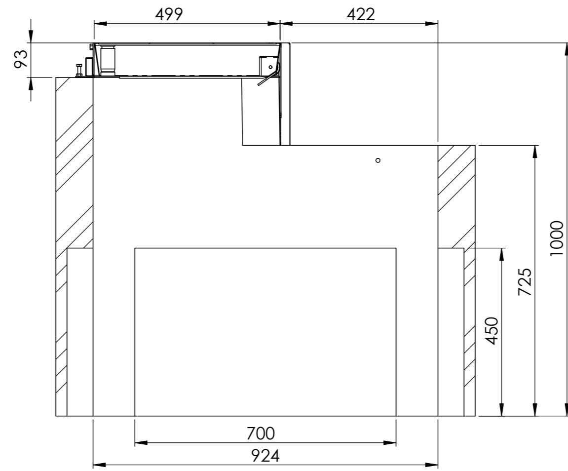
SCHNITT A-A
